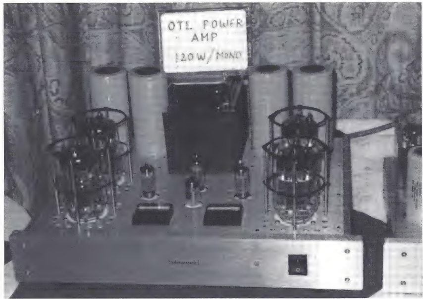
Een OTL van Silwaweld met 6C33's.
